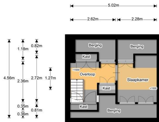
2e verdieping
