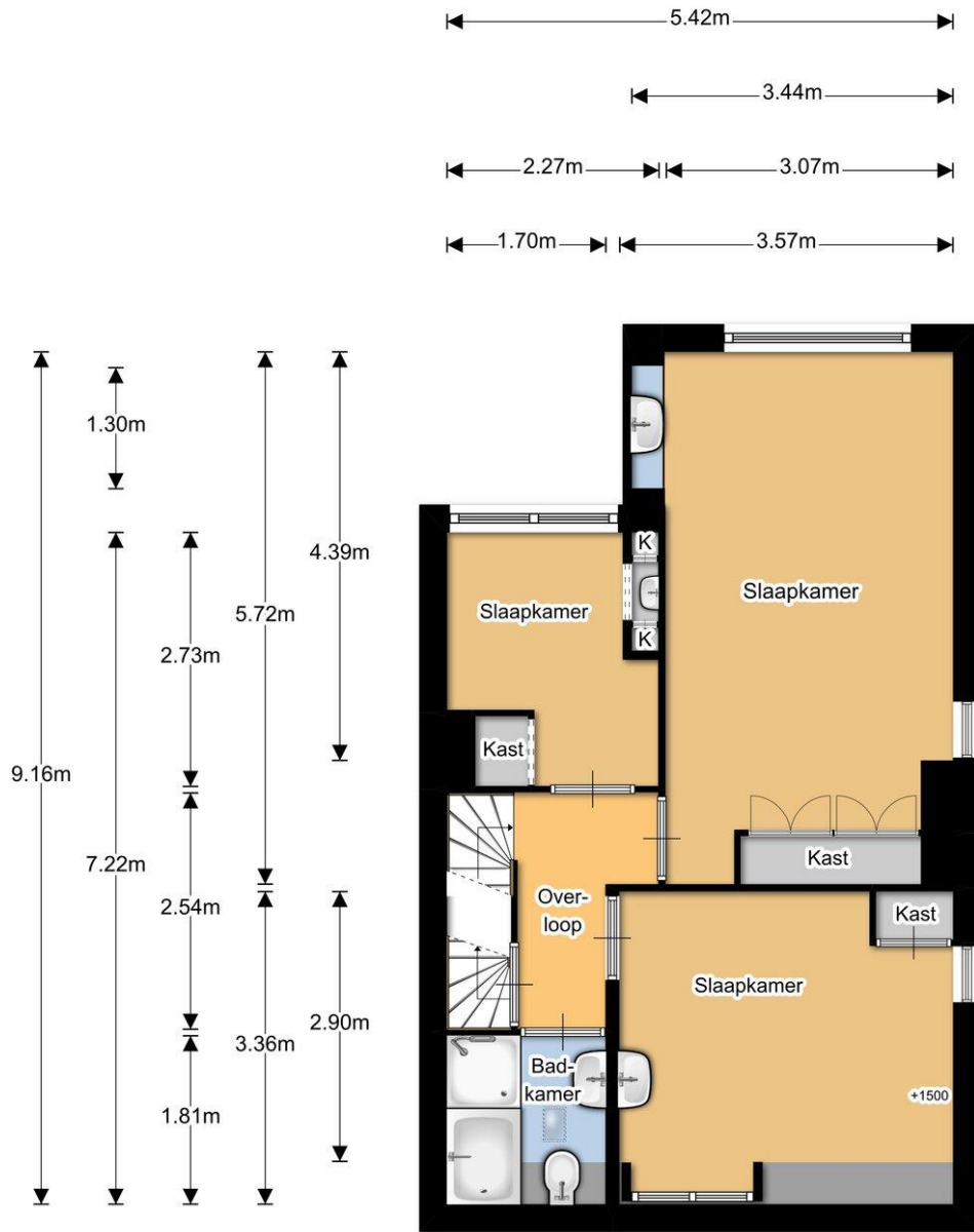
1e verdieping
