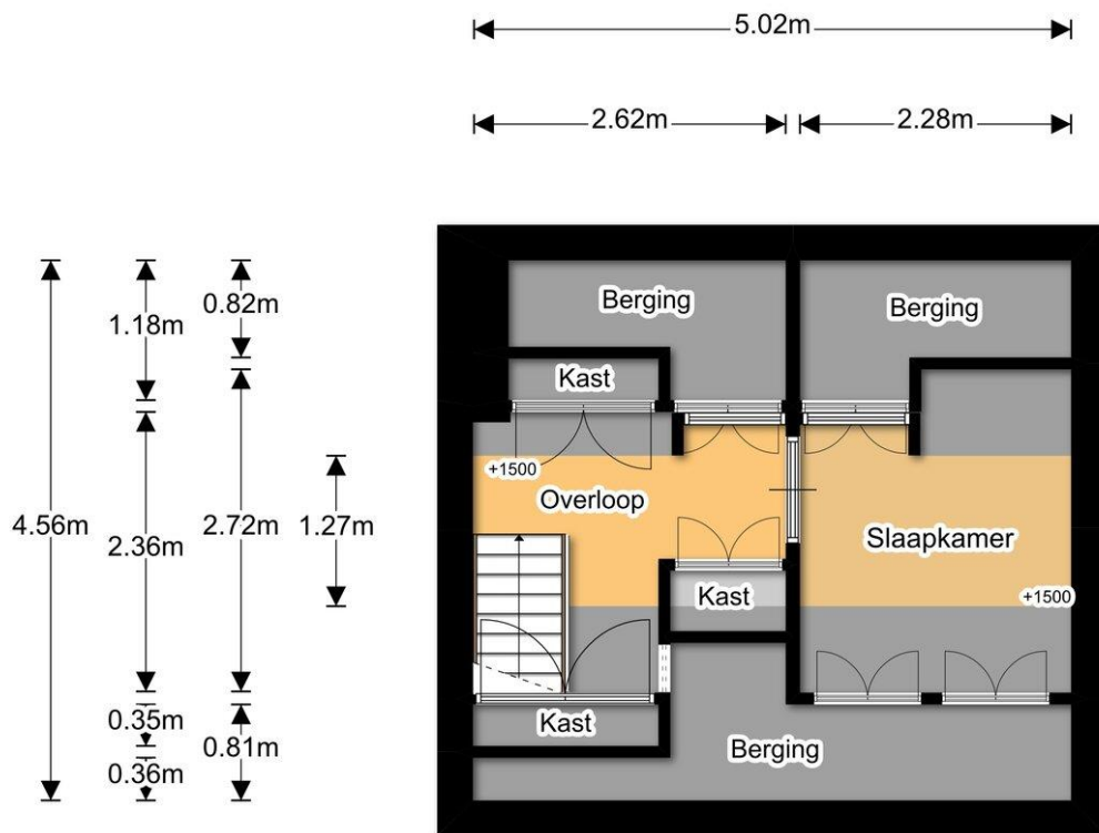
2e verdieping
