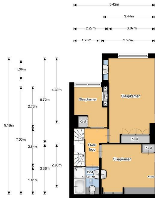
1e verdieping
