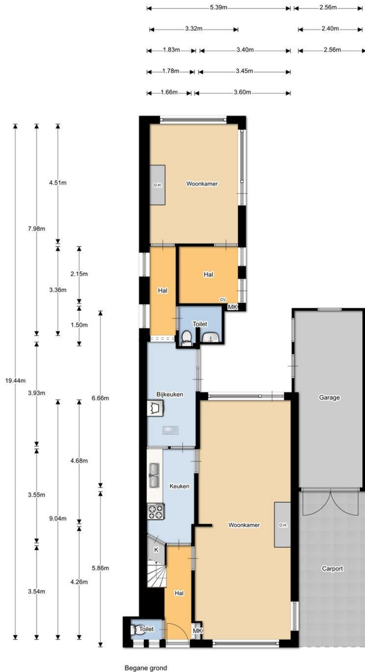
Begane grond
